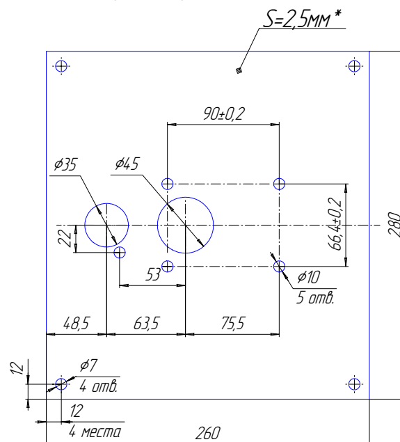
Рис 8.3- Пластина монтажная
